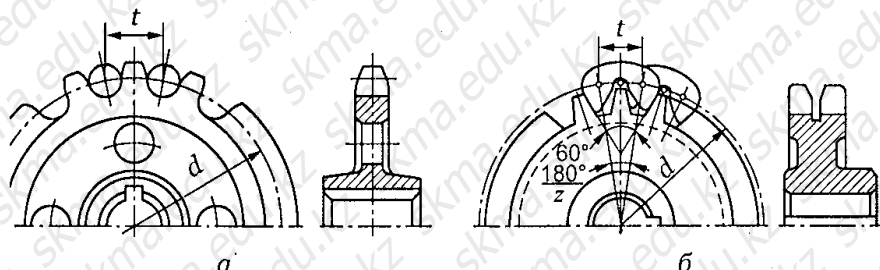
Рис. 10.2. Типы звездочек для цепных передач: а — для втулочной и роликовой цепи; б — для зубчатой цепи
